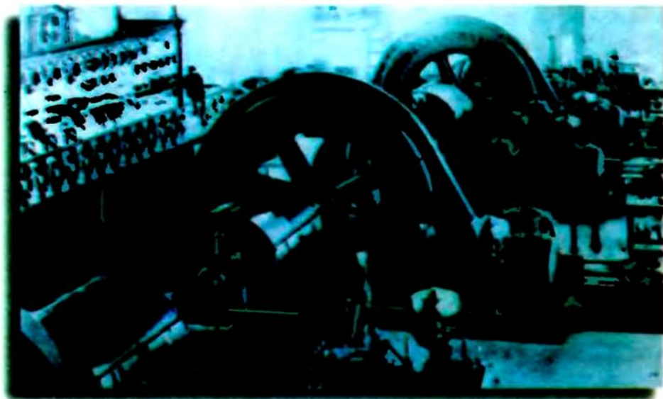
Друга електрична станція. Дніпровський завод (с. Кам'янське Катеринославської губернії). Поштівка
