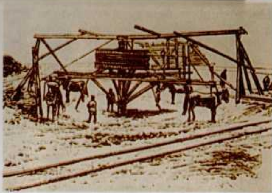
Кінний привід для підйому з шахти вагонеток з рудою. XIX ст.
