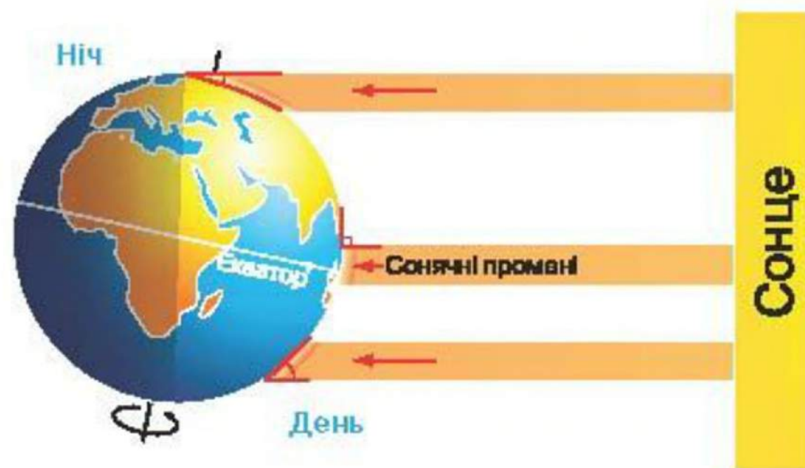
Схема добового обертання Землі
