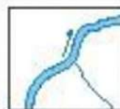
Річка. Напрямок течі
