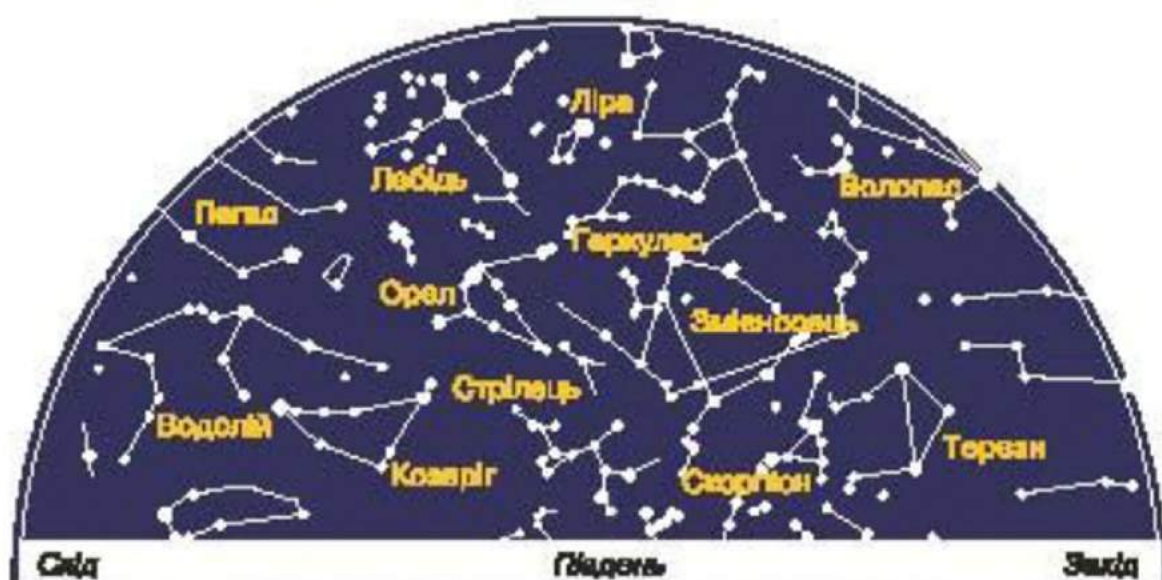
Карта зоряного неба влітку над Києвом
