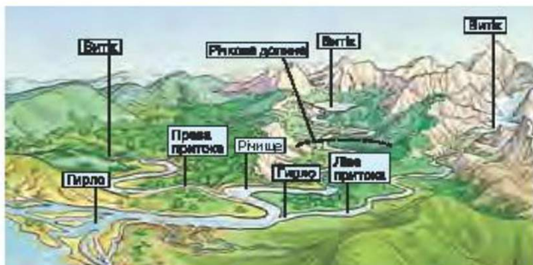
Схематичний малюнок будови річки
