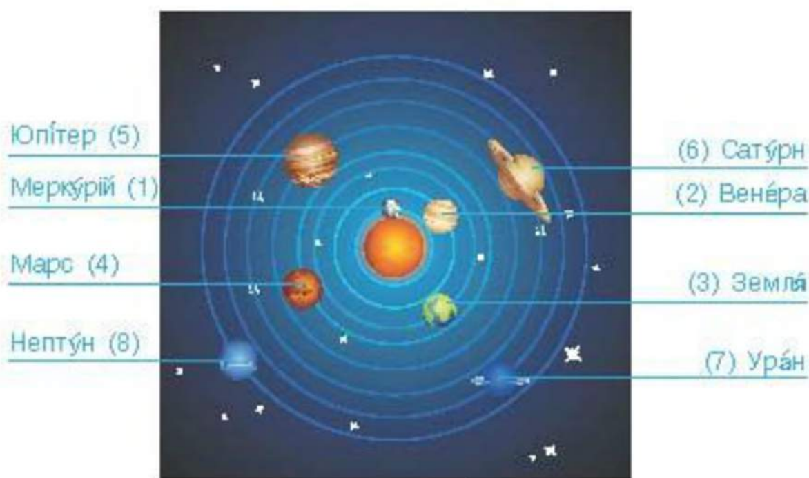
Схема будови Сонячної системи
