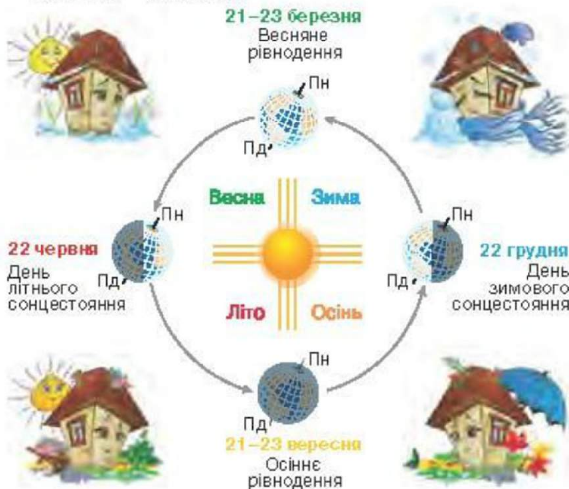
Схема річного руху Землі навколо Сонця
